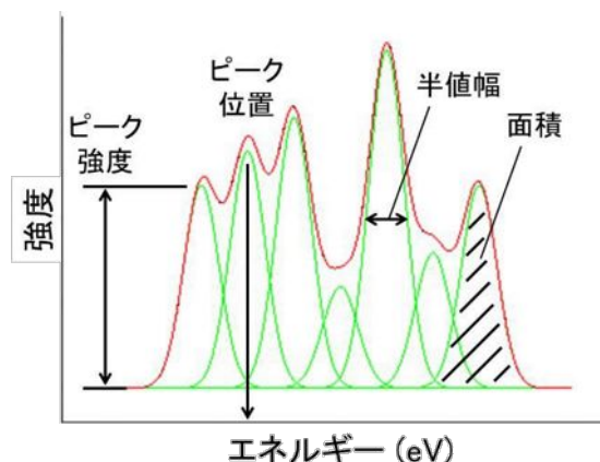
図2 価電子帯スペクトルの波形分離
