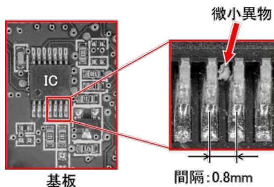
図1 プリント配線基板の微小異物の例
