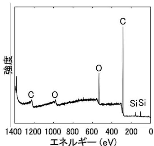
図3 不明異物のワイドスペクトル
